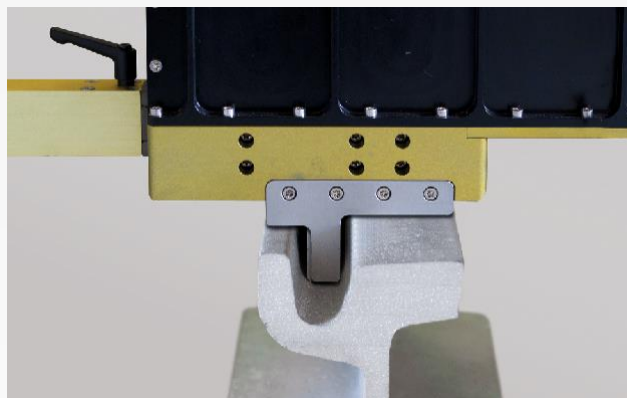
Měření drážkovaných kolejnic (volitelně)
